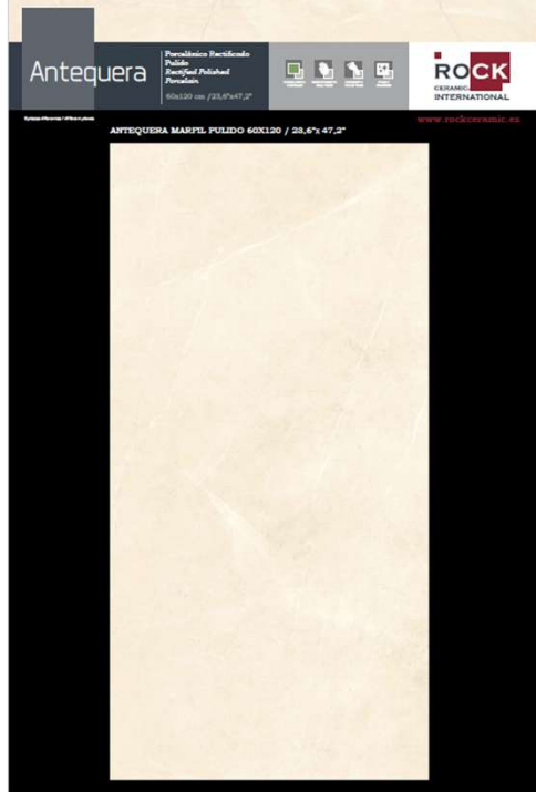
RC-634 ANTEQUERA MARFIL PL 60X120 1925x1005x13 Code: 036963 Antequera Marfil Pulido 60x120 (1pc) Weight: 30,00Kgs Price: E10- 60,00€
